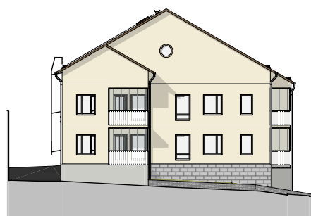
JULKISIVU LÄNTEEN
