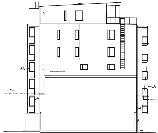
JULKISIVU KOILLISEEN
