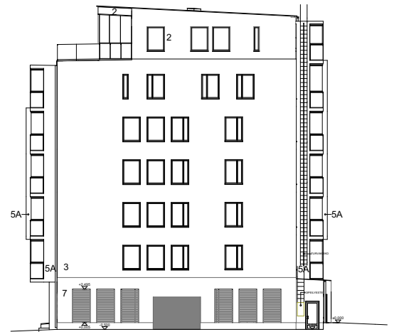
JULKISIVU LOUNAASEEN
